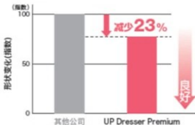
形状变化比较 (修整器起伏)
