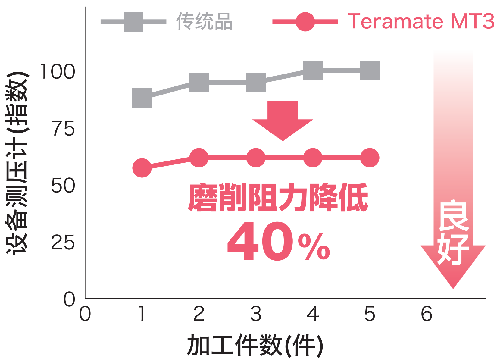
磨削阻力比较
