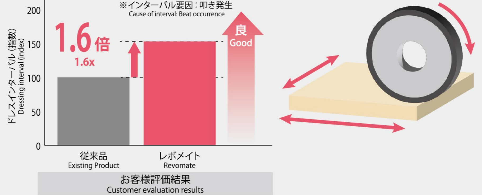
ドレスインターバル比較 Dressing interval comparison
